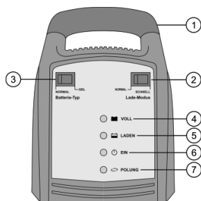
Figura 1: Vista della parte anteriore
