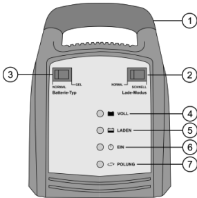
Bild 1: Ansicht Vorderseite
