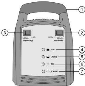
Afbeelding 1: voorzijde
