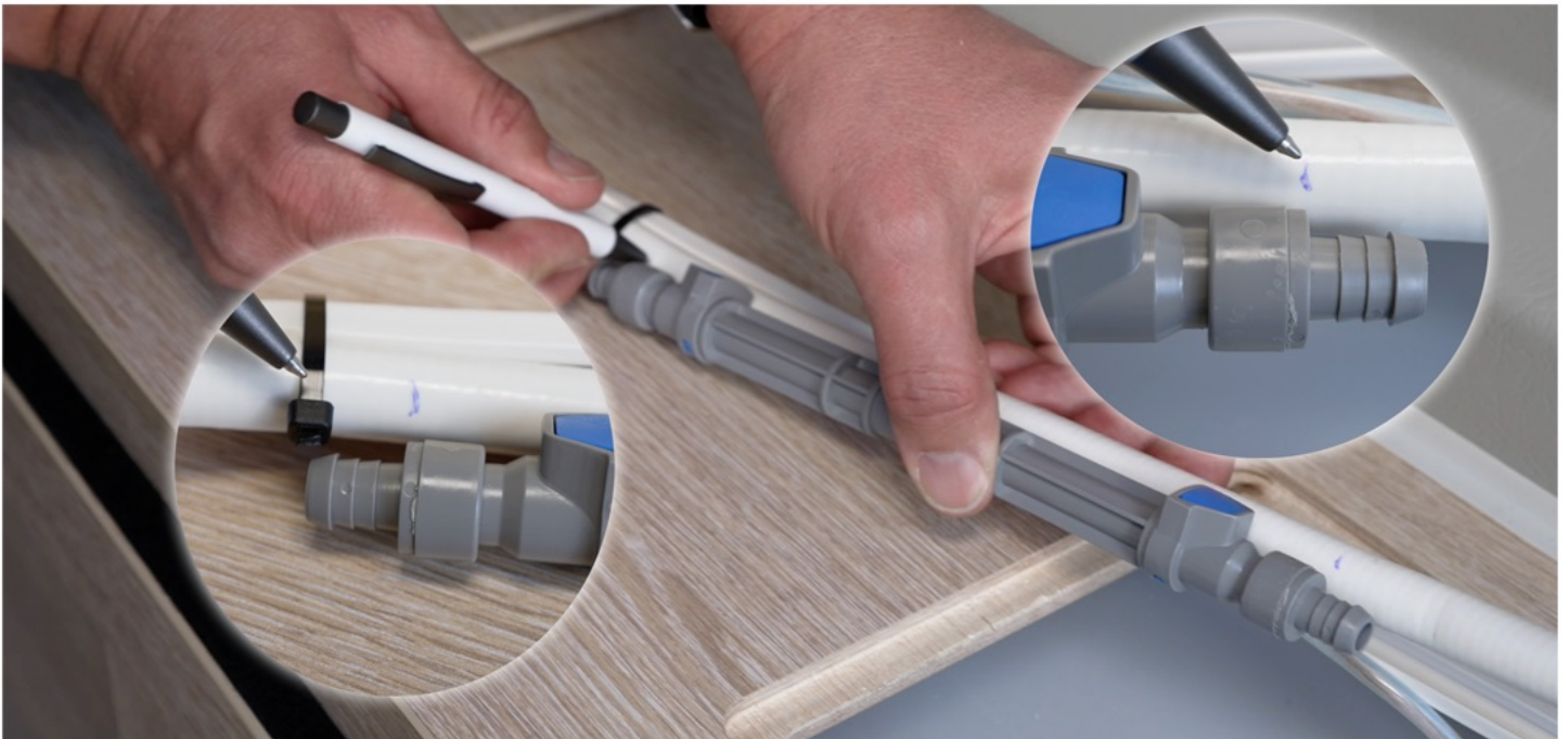
Abbildung 3: Markieren des zu setzenden Schnittes am Wasserschlauch
