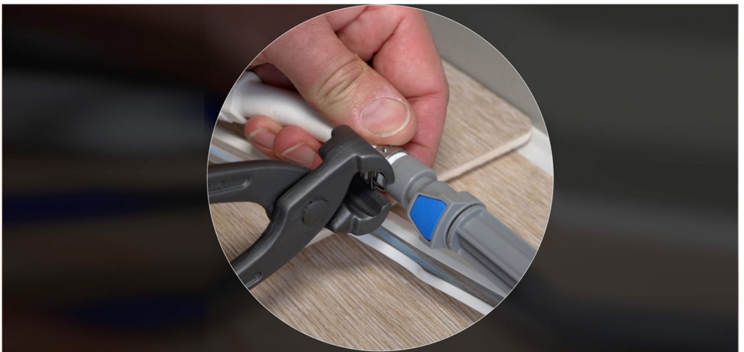
Abbildung 5: Schlauchschellen aufschieben, Click-and-Ready-Anmschlüsse einsetzen und verkrumpfen..
