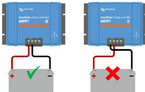
Beispiele für richtige und falsche (vertauschte) Batteriepolartät.
