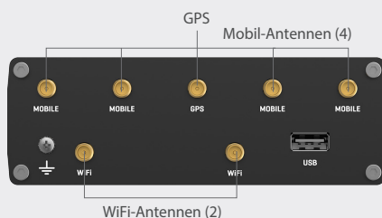
Rückansicht
